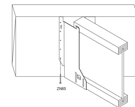
取付図
