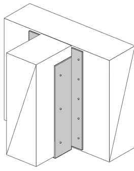
取付図
