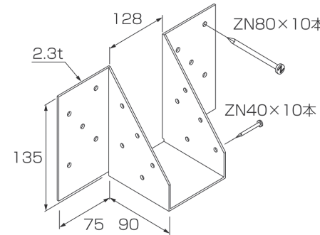
取付図
