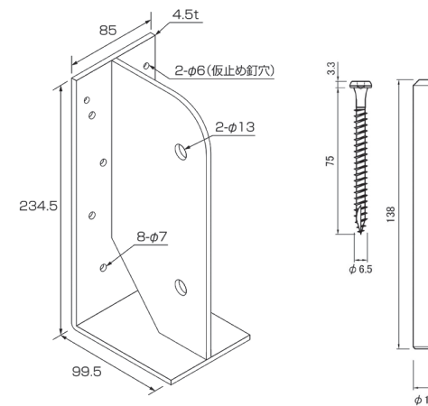
金物図
