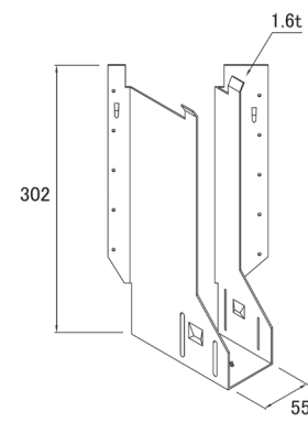
取付図
