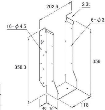
金物図
