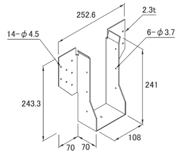
金物図
