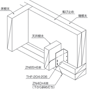
取付図
