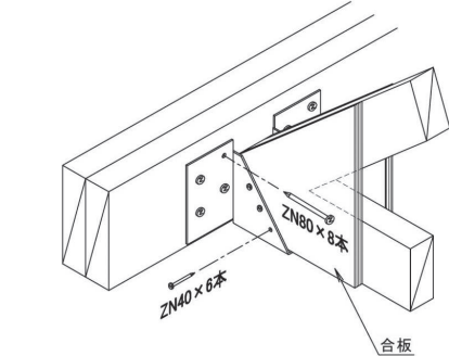
取付図
