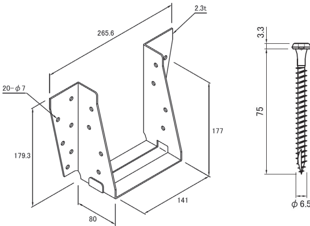
金物図
