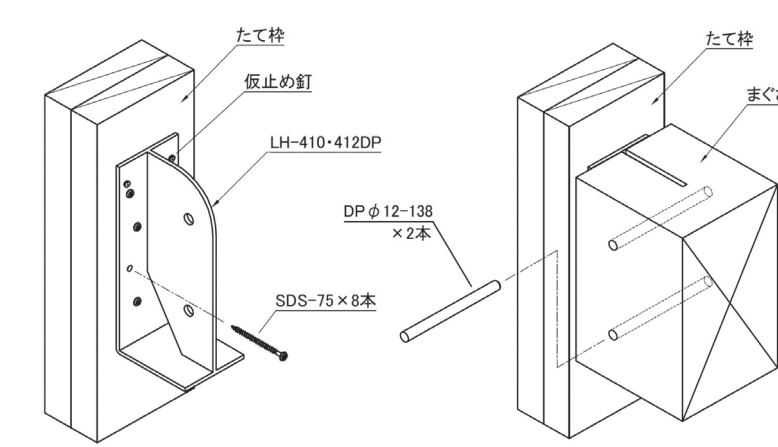
取付図
