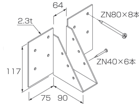
金物図
