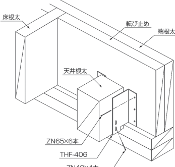
取付図
