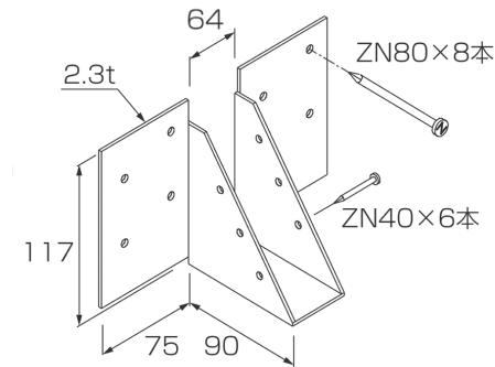
金物図
