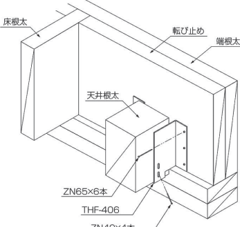
取付図
