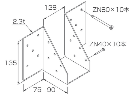
取付図
