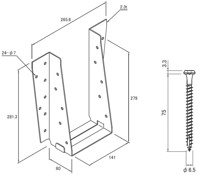
金物図
