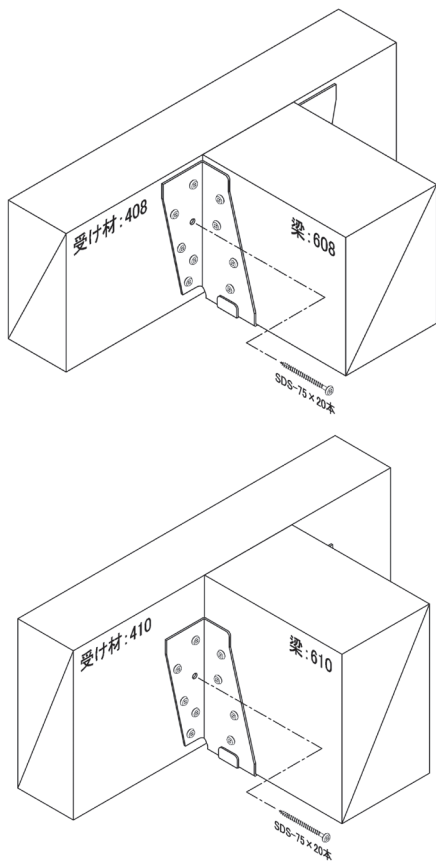
取付図
