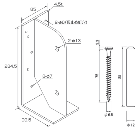
金物図
