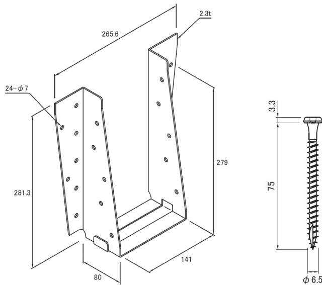
金物図
