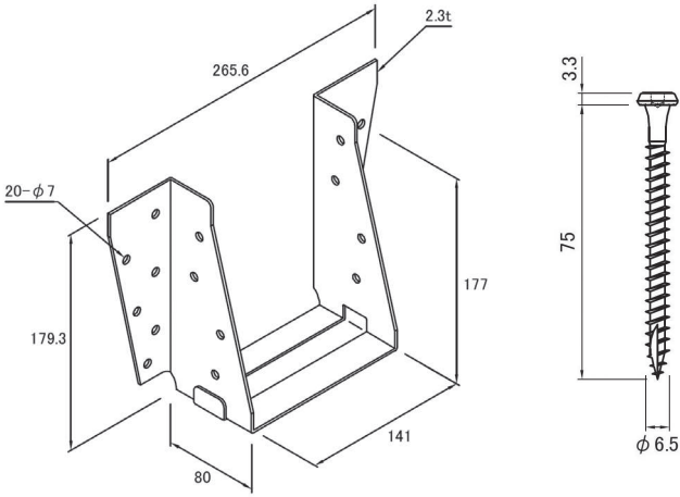
金物図
