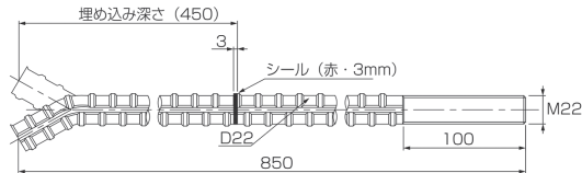
金物図
