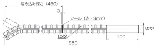
金物図
