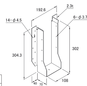
金物図
