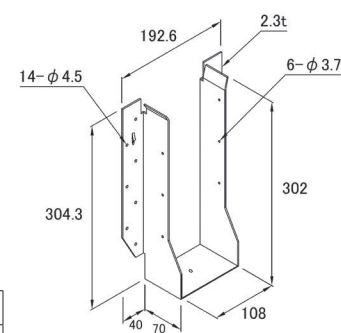
金物図
