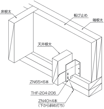
取付図
