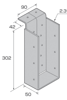
取付図
