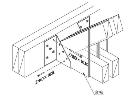
取付図
