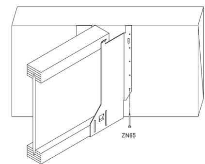
取付図
