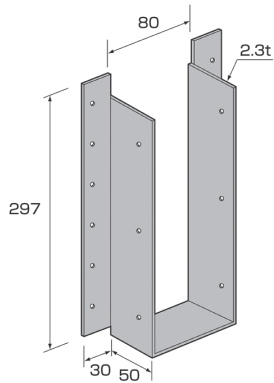
取付図
