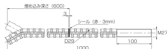
金物図
